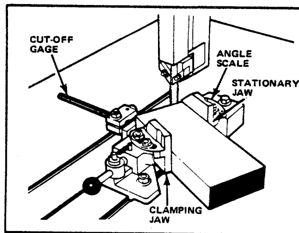
FIG. 31. UNIVERSAL VISE.
